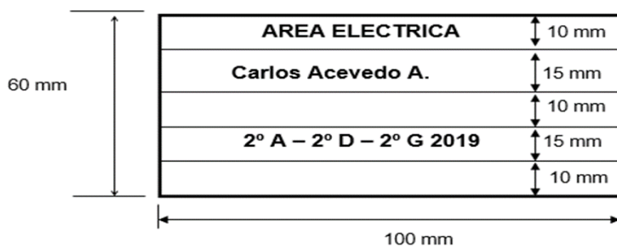
EJEMPLO DE PARCHE PARA EL SLACK (Bordado con hilo rojo)
